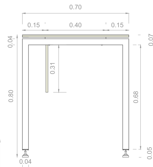
VISTA LATERAL
