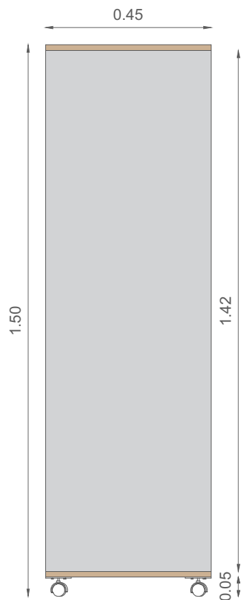
VISTA LATERAL
