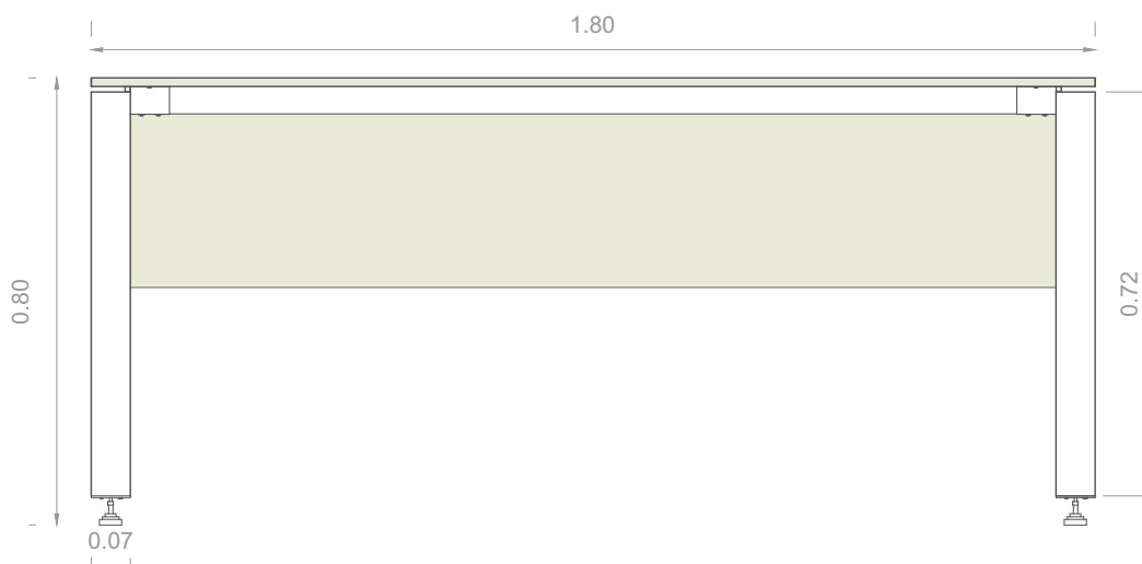
VISTA POSTERIOR
